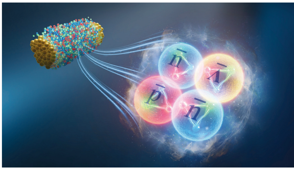
重离子碰撞产生反物质超核-4艺术图。(中国科学院近代物理研究所提供)
