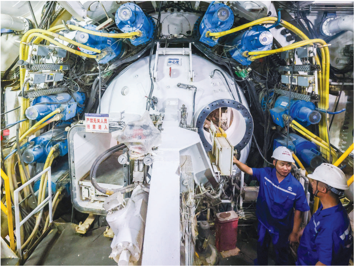
3月15日,由中铁十四局施工的广州至湛江高速铁路湛江湾海底隧道顺利贯通。该隧道由一台直径14.33米的盾构机掘进,历时33个月,掘进7551米,是目前国内独头掘进距离最长的穿海高铁盾构隧道。图为技术员在广湛高铁湛江湾海底隧道盾构机内检查设备工作状态。
