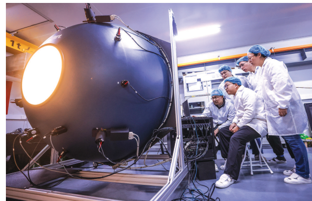
中科院上海技术物理研究所温室气体载荷团队成员正在进行利用积分球模拟太阳光的真空光校测试。 本报记者 袁婧媛
