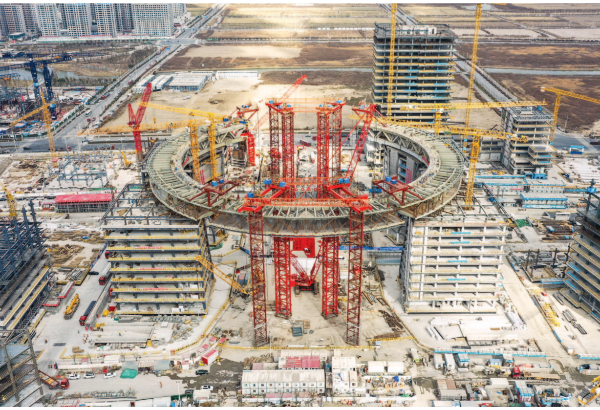
“荣耀之环”起吊合龙仪式现场。
