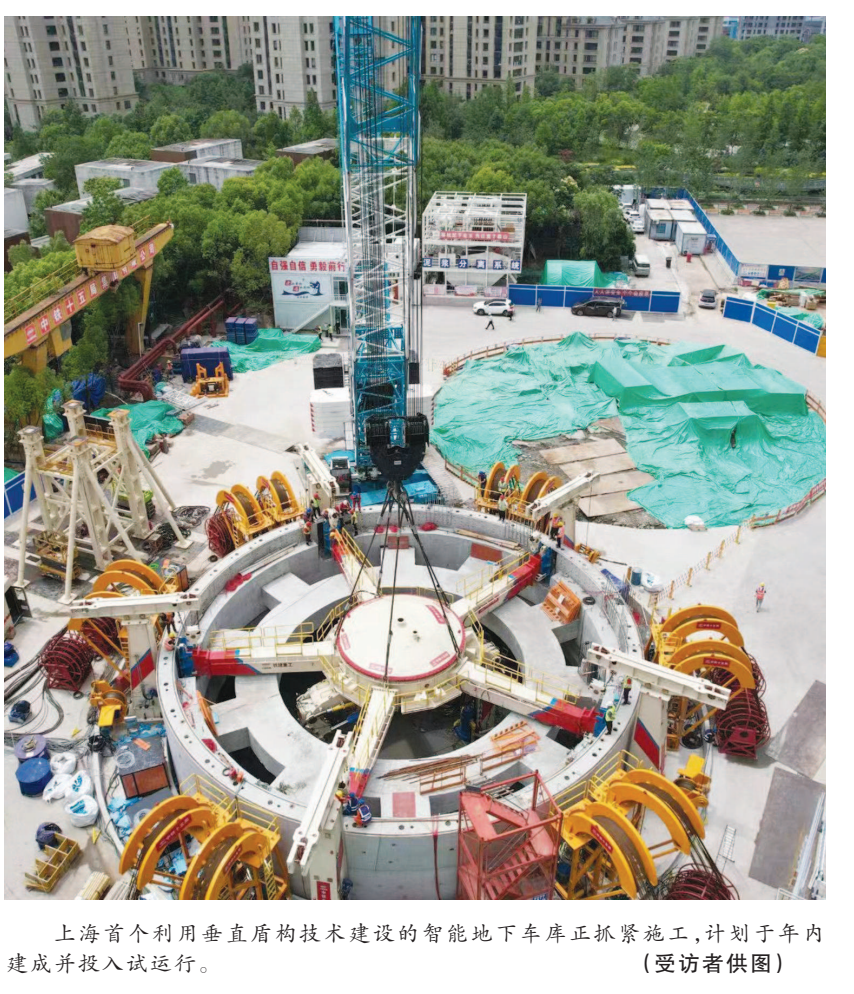
上海首个利用垂直盾构技术建设的智能地下车库正抓紧施工,计划于年内建成并投入试运行。
