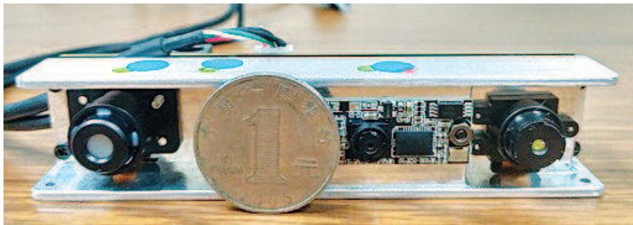
基于第一代三维深度感知专用芯片研制的“中距离 3D 深度相机”。(西安交大供图)
