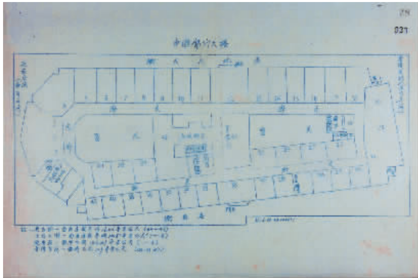
中汇银行大楼平面图（上海博物馆 1959 年档案材料）
