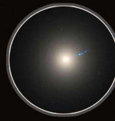
哈勃太空望远镜拍摄的M87
