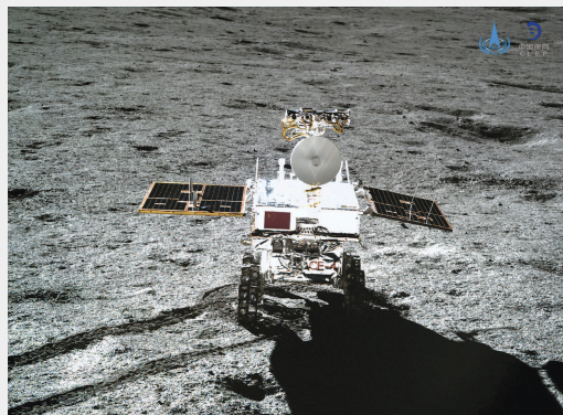
嫦娥四号着陆器地形地貌相机对玉兔二号巡视器成像。
