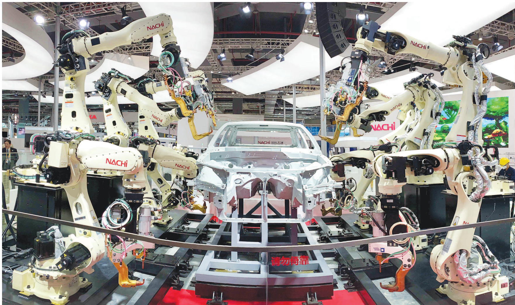
在专家的调试下, 日本不二越公司的高密度汽车点焊机械臂已做好展出准备。
