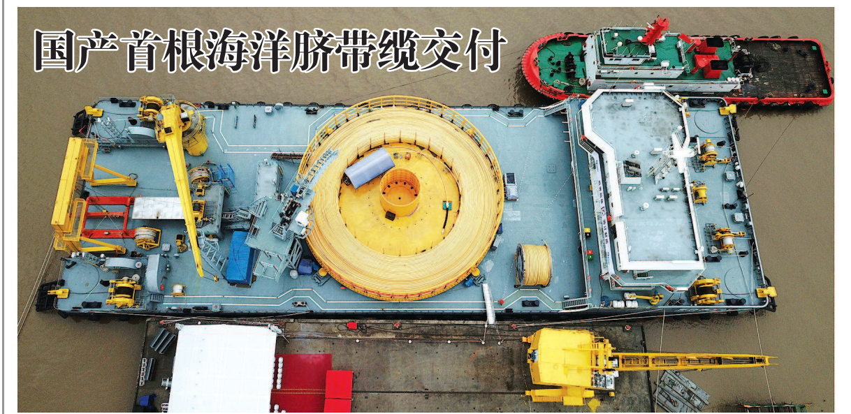
6月20日，由我国自主研发、设计、制造的首根国产化海洋脐带缆在浙江省宁波市北仑区东方电缆码头交付...
